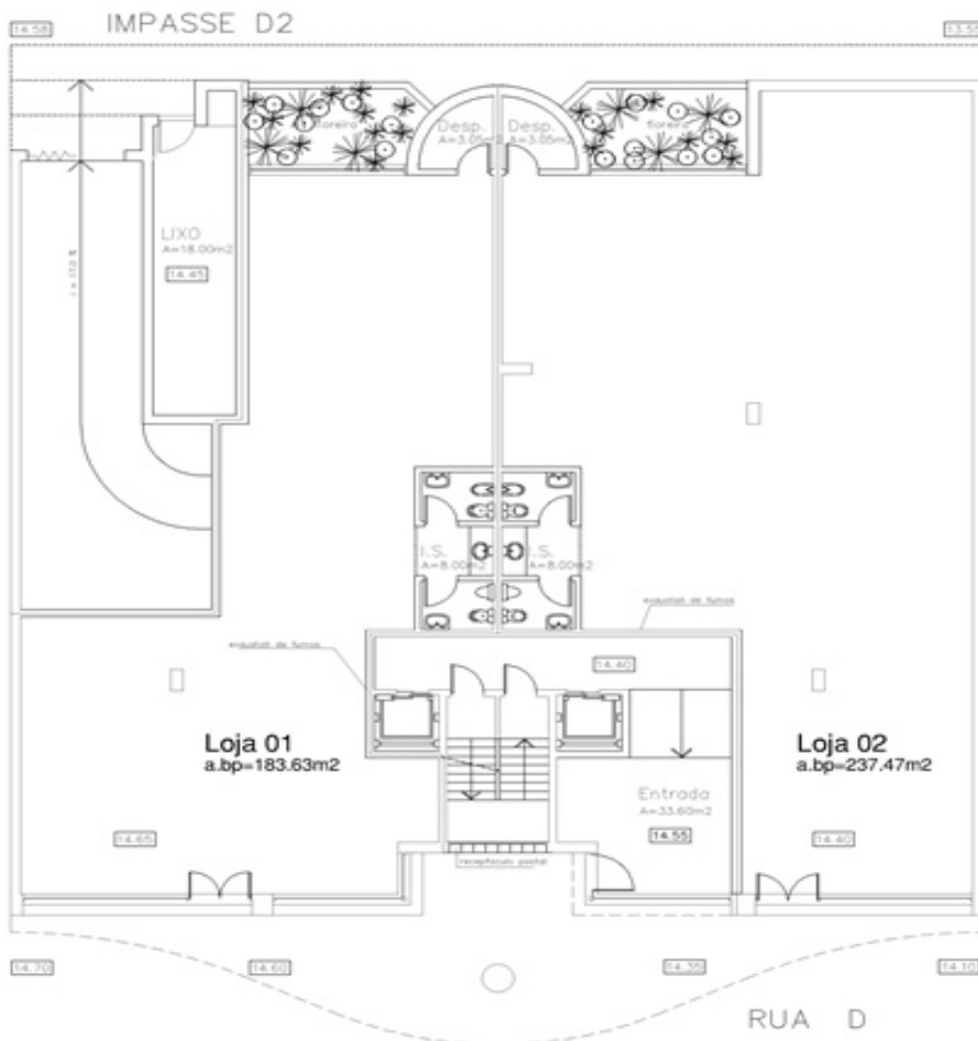
Planta piso 0
