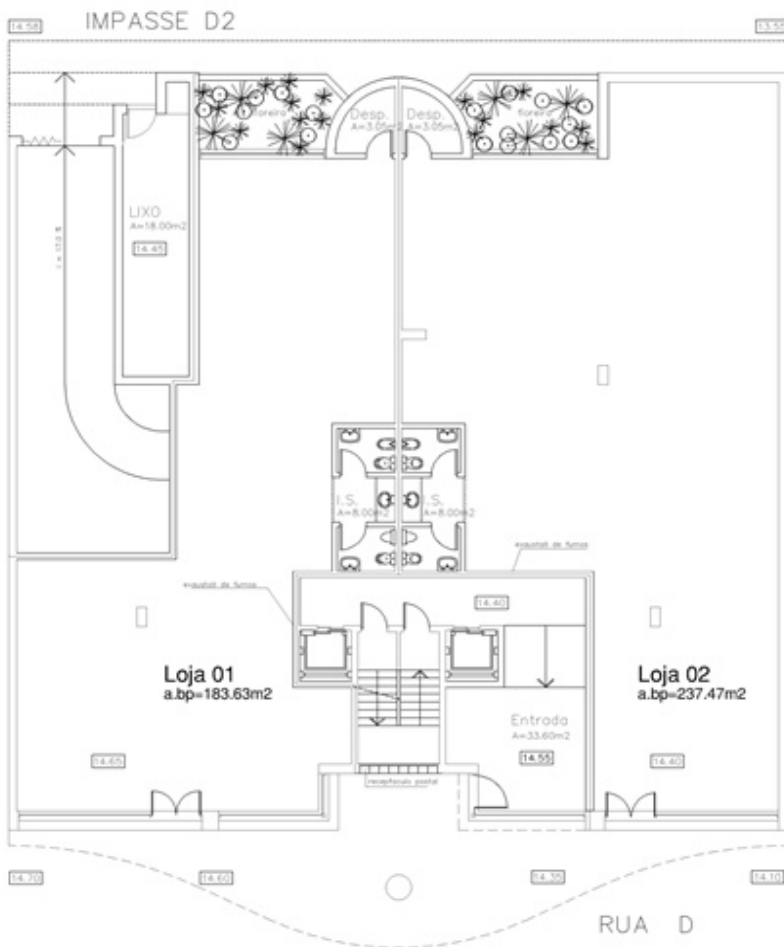
Planta piso 0
